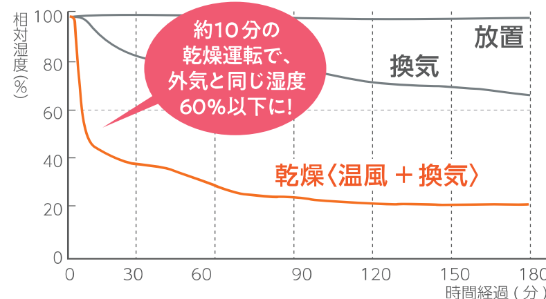
■浴室湿度の変化
