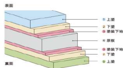
ニスクカラーProの塗膜の構成
